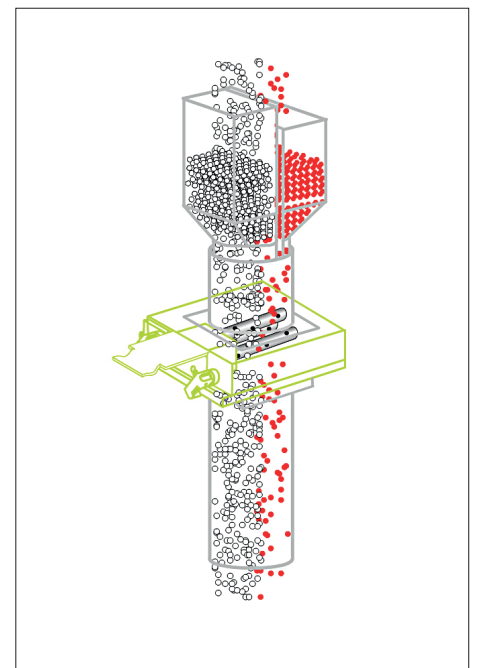
Der Rohr-Magnet SAFEMAG wird in stehenden oder langsam fließenden Materialsäulen eingesetzt.
